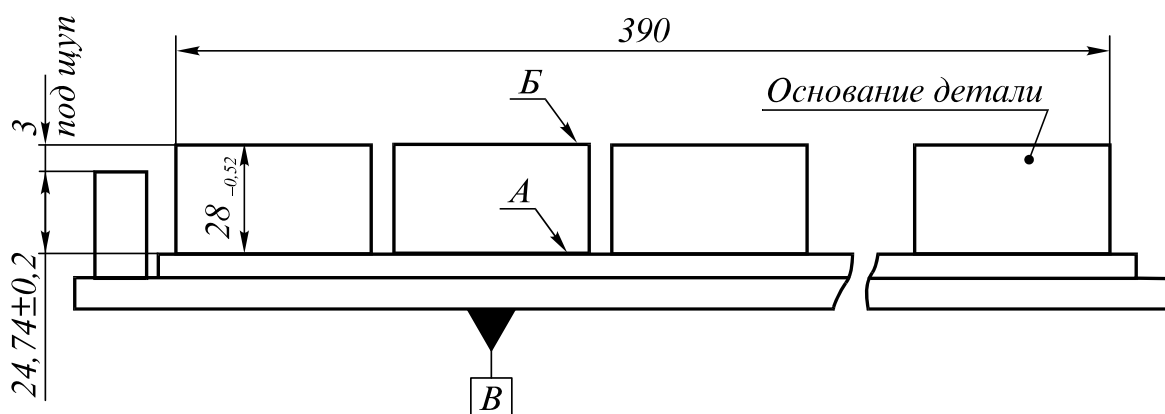
Рисунок 4.1 – Схема расчета точности приспособления
