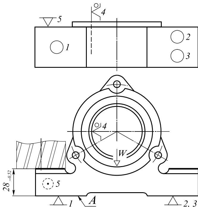
Рисунок 3.1 – Схема установки обрабатываемой детали
